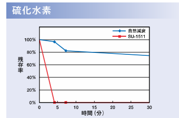
タバコの3大臭気成分といわれるアンモニア、アセトアルデヒド、硫化水素を急速に脱臭します。(試験条件:4m 3 のステンレス製無臭室にて各臭気成分を揮発し残存率を検知管にて測定。SU-1511運転時の値は、強力脱臭フィルターを装着した場合。)
